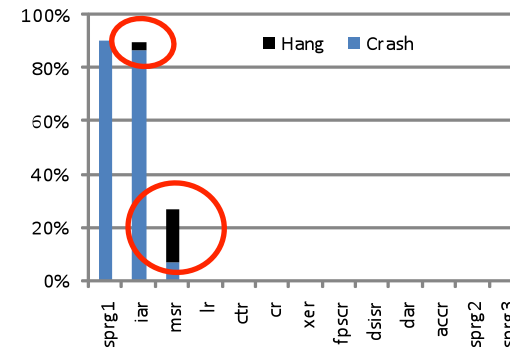
AIX System
